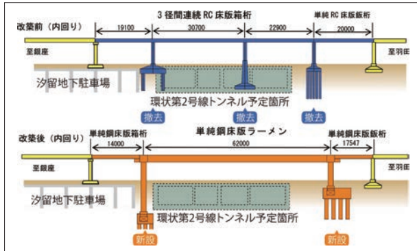
首都高速汐留高架橋 橋梁断面図
