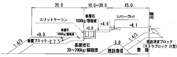
面的防護方式の標準断面図
