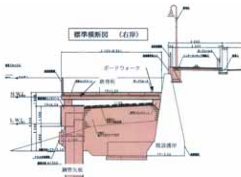
標準横断面図
